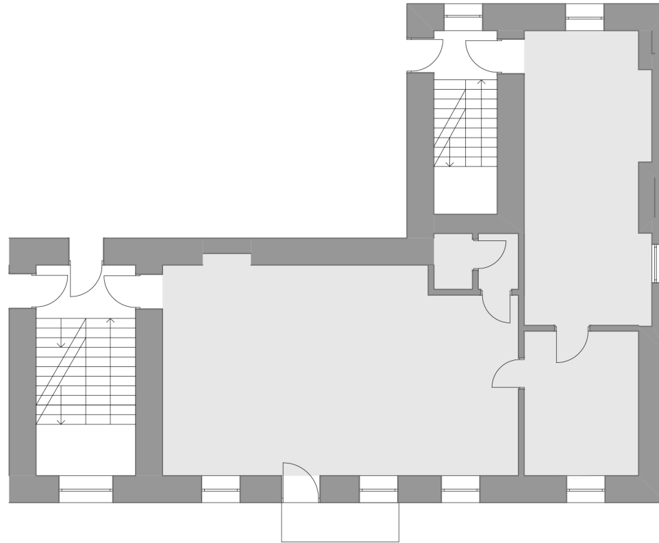
План приміщення Площа приміщення 91,1 м 2
